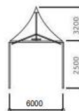
6x6m Perfil 65x65x3 mm
