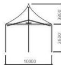
10x10m Perfil 122x68x3 mm
