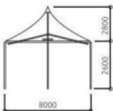
8x8m Perfil 122x68x3 mm
